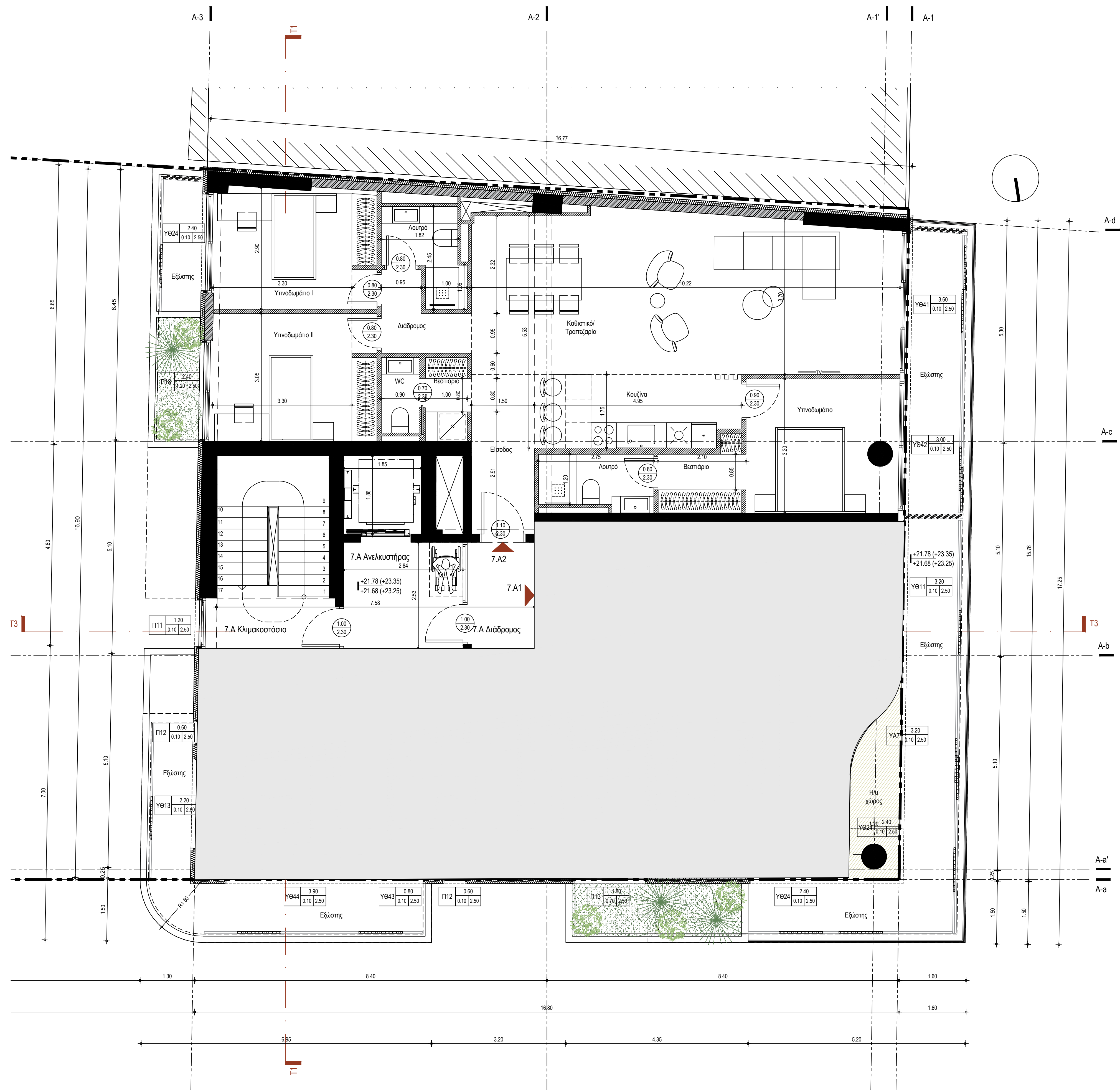
ΚΤΙΡΙΟ Α ΚΑΤΟΨΗ 7ου ΟΡΟΦΟΥ ΚΛΙΜΑΚΑ 1:100
