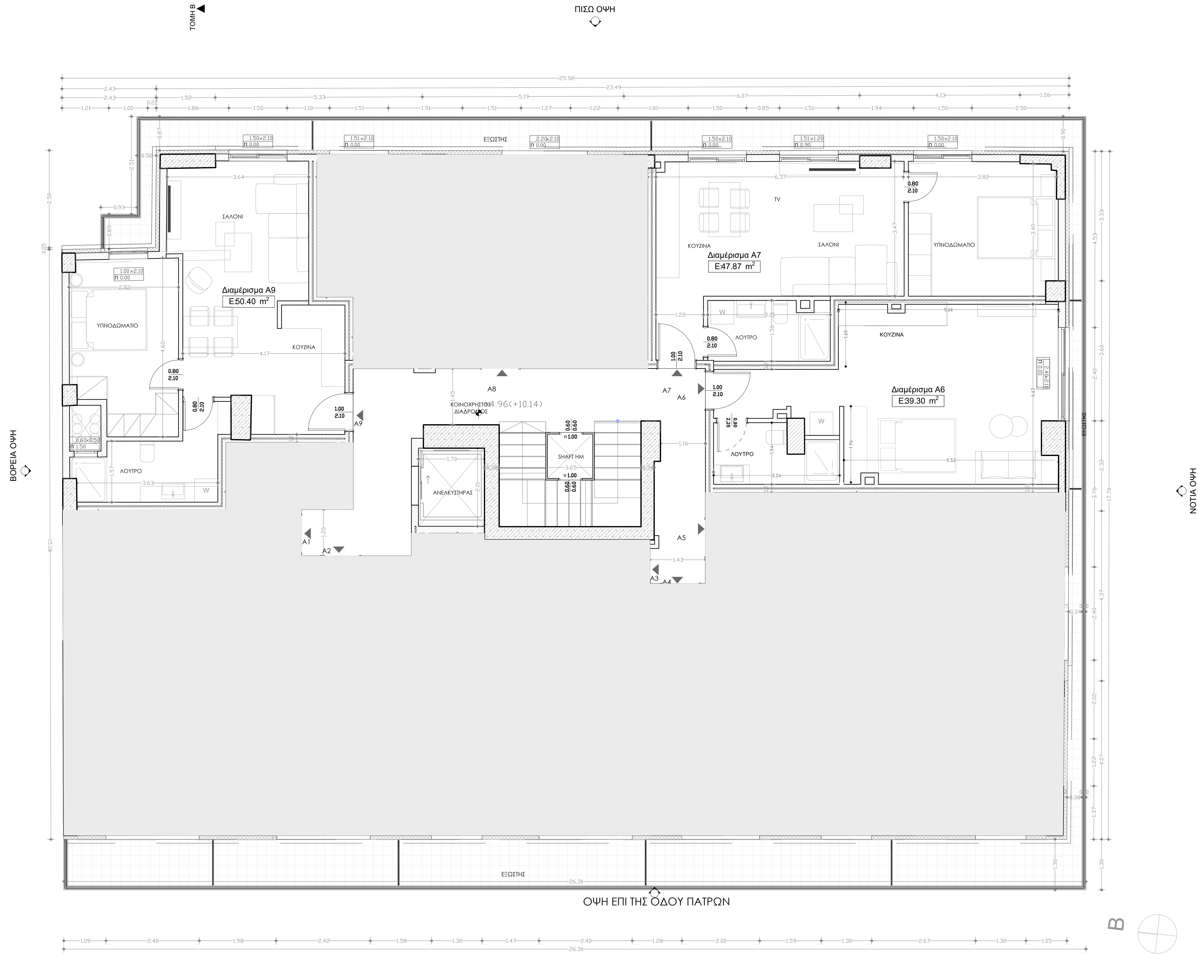
ΚΑΤΟΨΗ 1ου ΟΡΟΦΟΥ ΚΛΙΜΑΚΑ 1:100
