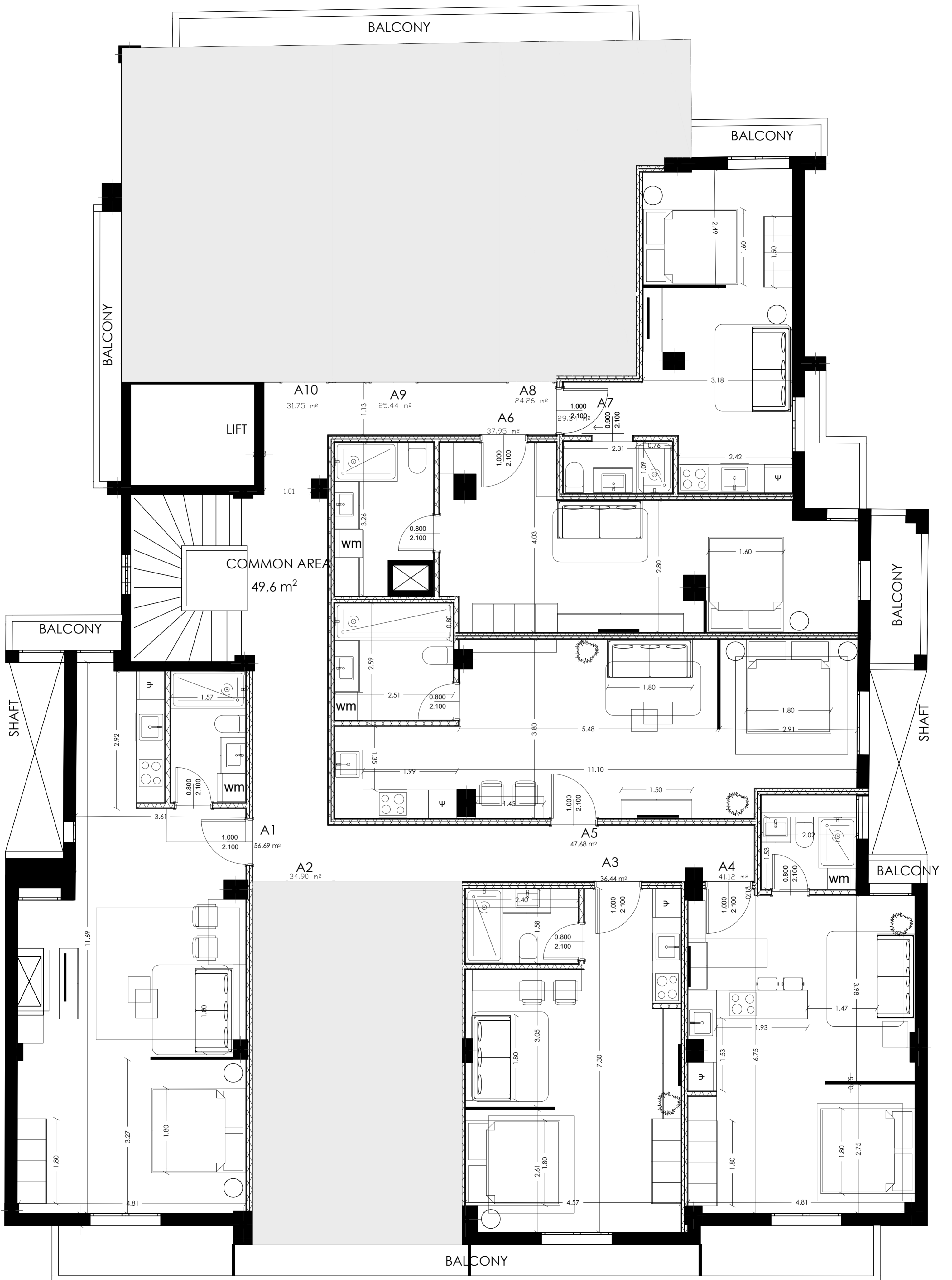
ΚΑΤΟΨΗ 4ου ΟΡΟΦΟΥ ΚΛΙΜΑΚΑ 1:50
