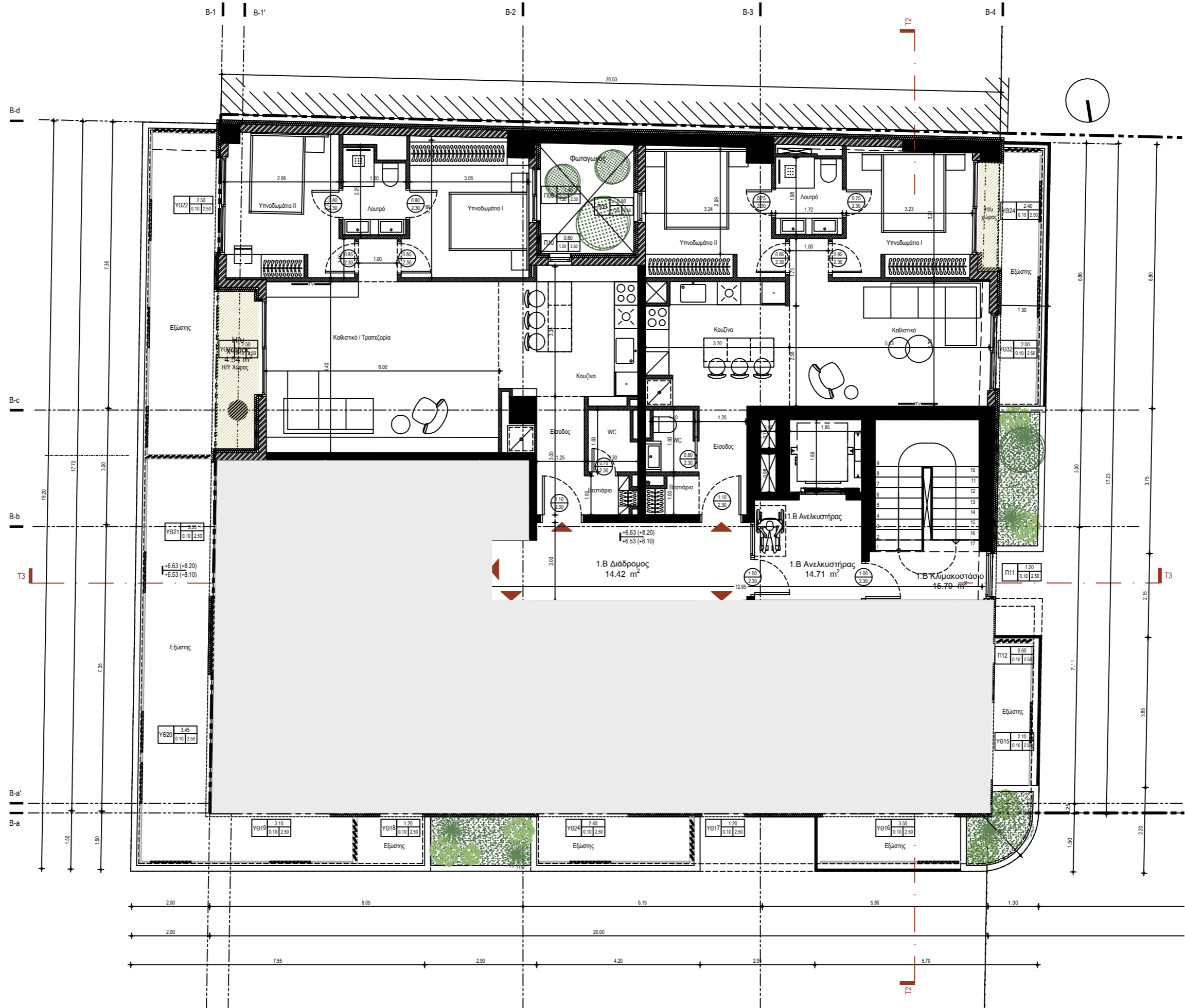
ΚΤΙΡΙΟ Β ΚΑΤΟΨΗ 2ου ΟΡΟΦΟΥ ΚΛΙΜΑΚΑ 1:100
