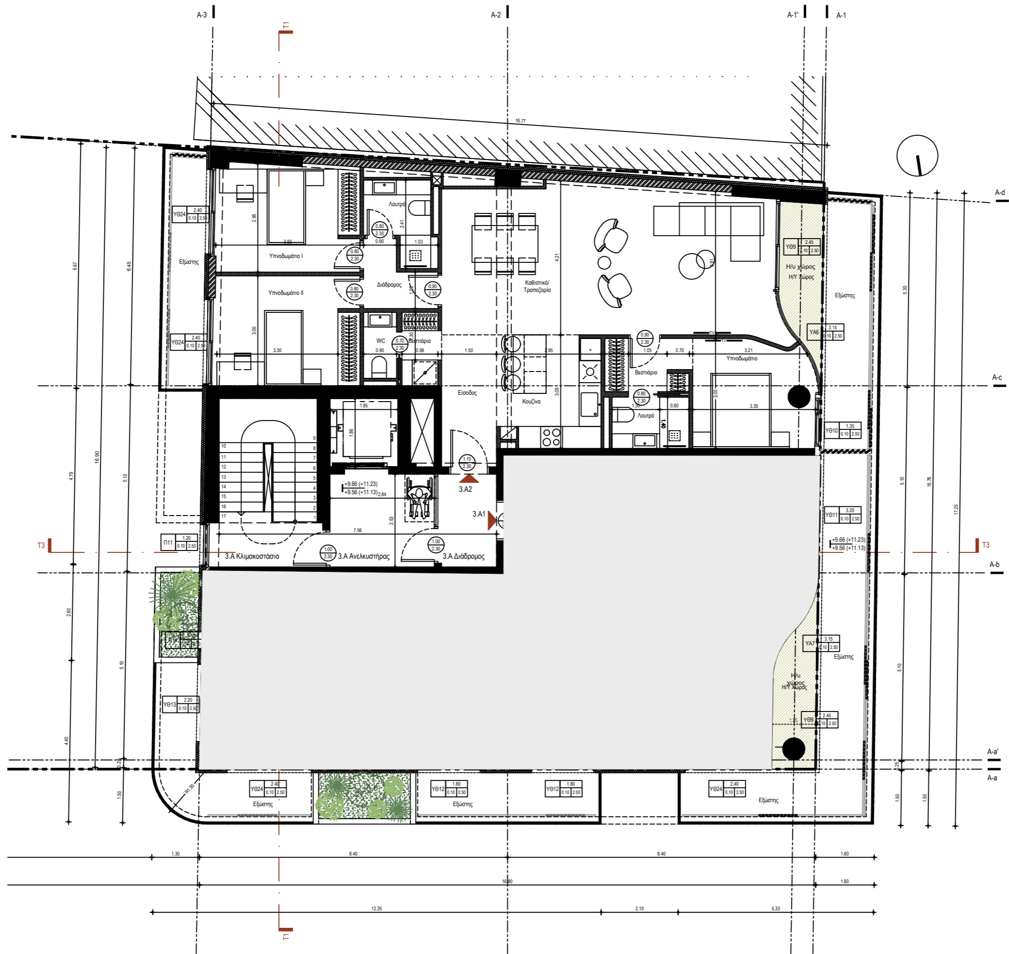
ΚΤΙΡΙΟ Α ΚΑΤΟΨΗ 3ου ΟΡΟΦΟΥ ΚΛΙΜΑΚΑ 1:100
