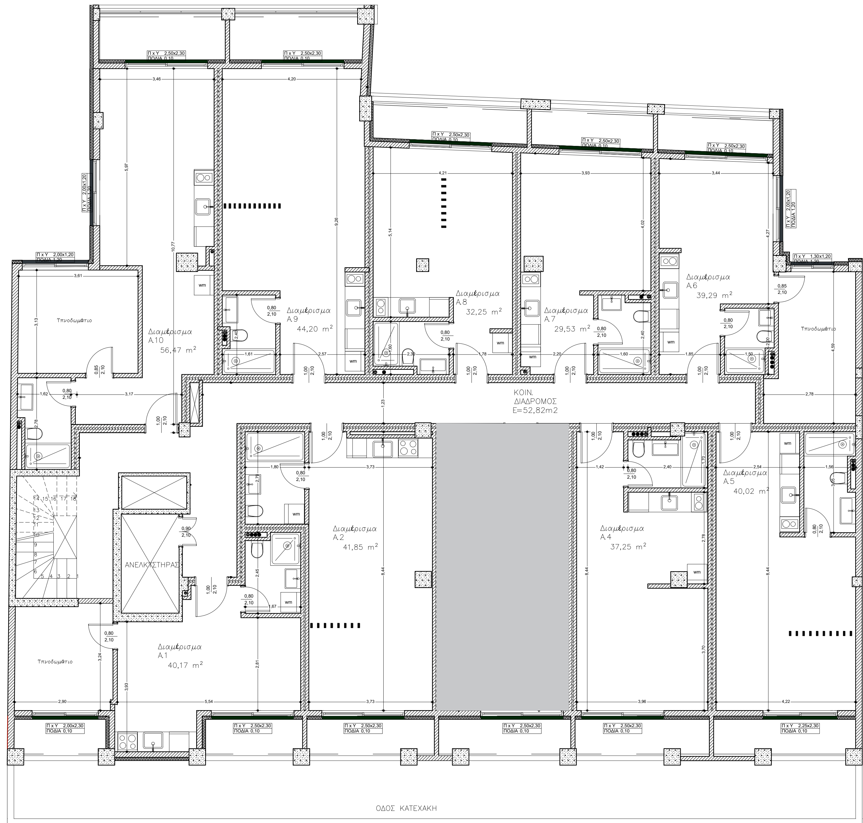
ΚΑΤΟΨΗ 1ου ΟΡΟΦΟΥ ΚΛΙΜΑΚΑ 1/100
